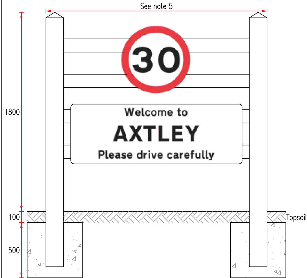
ELEVATION
